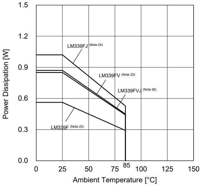
(e) LM339xxx
