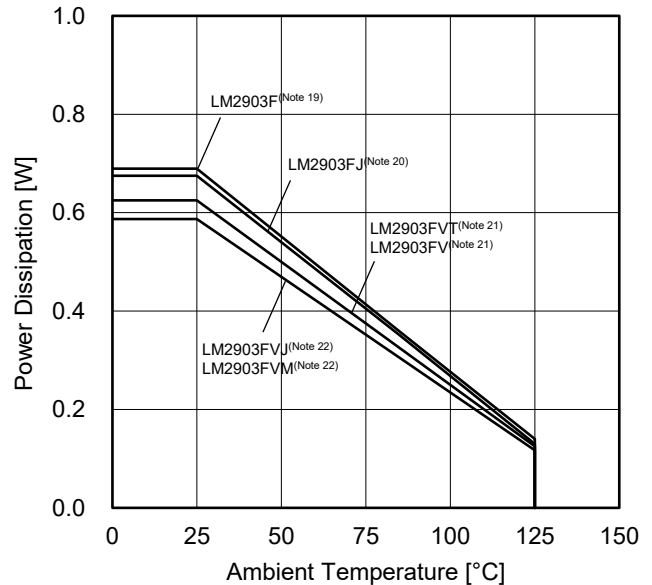
(d) LM2903xxx
