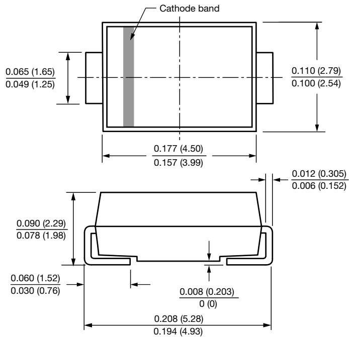
DO-214AC (SMA)
